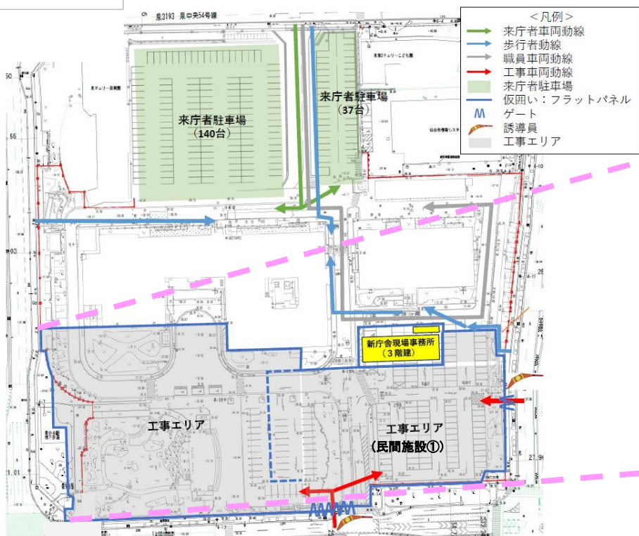
仮設計画図
