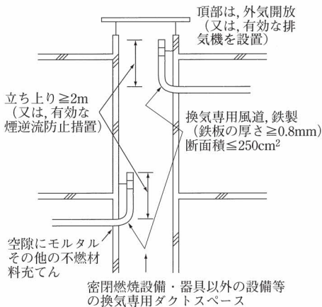
4.1 図2 換気専用ダクトスペースの場合
