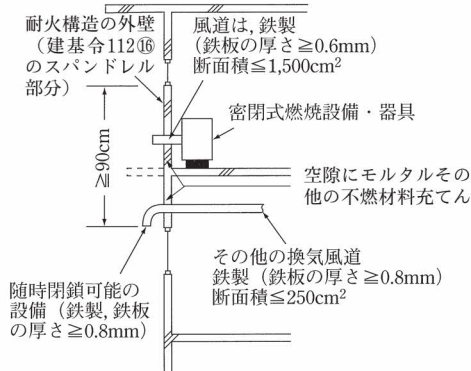
4.1 図3 耐火構造等の外壁(防火区画)を貫通する場合
