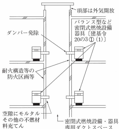
4.1 図1 密閉式燃焼設備・器具専用ダクトスペースの場合
