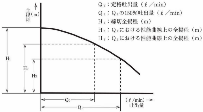
2.3 図1 揚程曲線図
