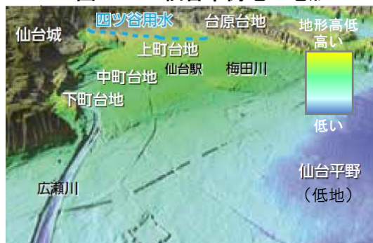
図 2-12 仙台市街地の地形
