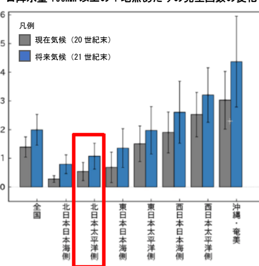
図 2-48 大雨等の年間発生回数の変化
