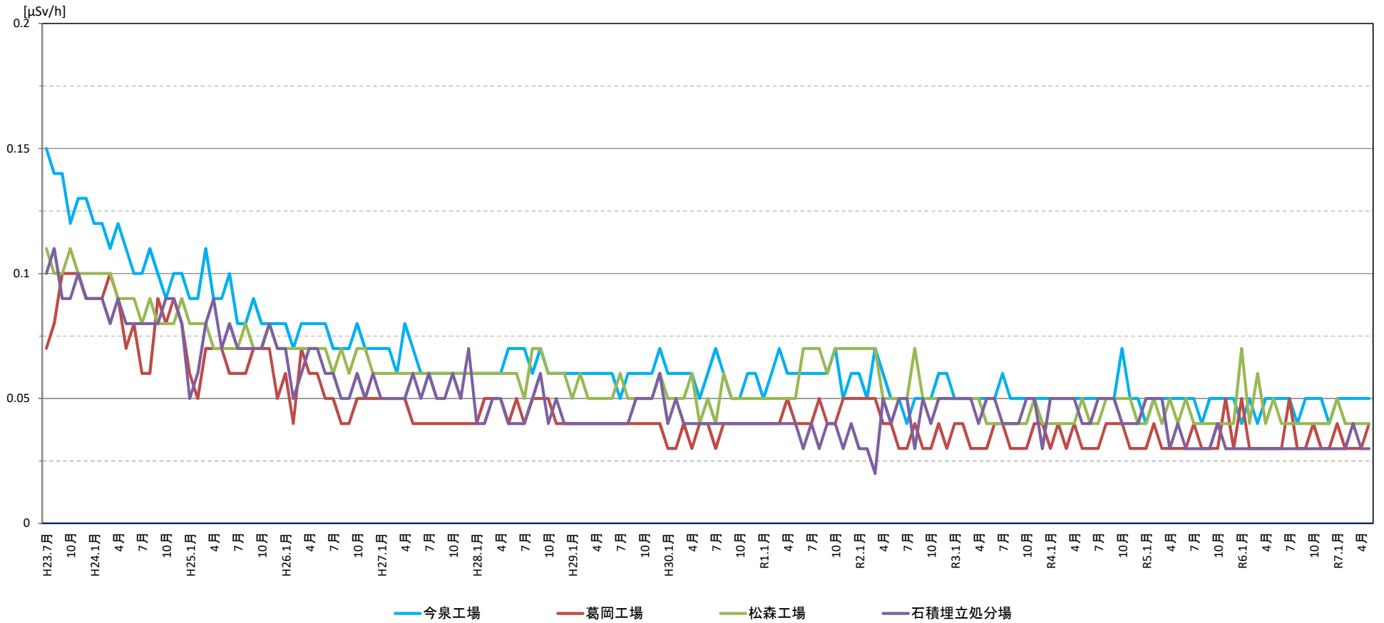
空間放射線量(敷地境界の最大値)の推移 (H23.7～R7.5)
