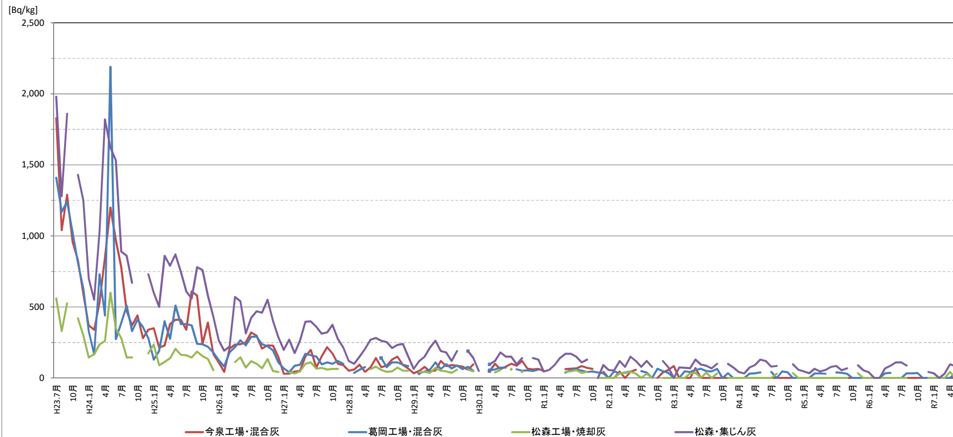
灰の放射性物質濃度の推移（H23.7～ R7.5）
