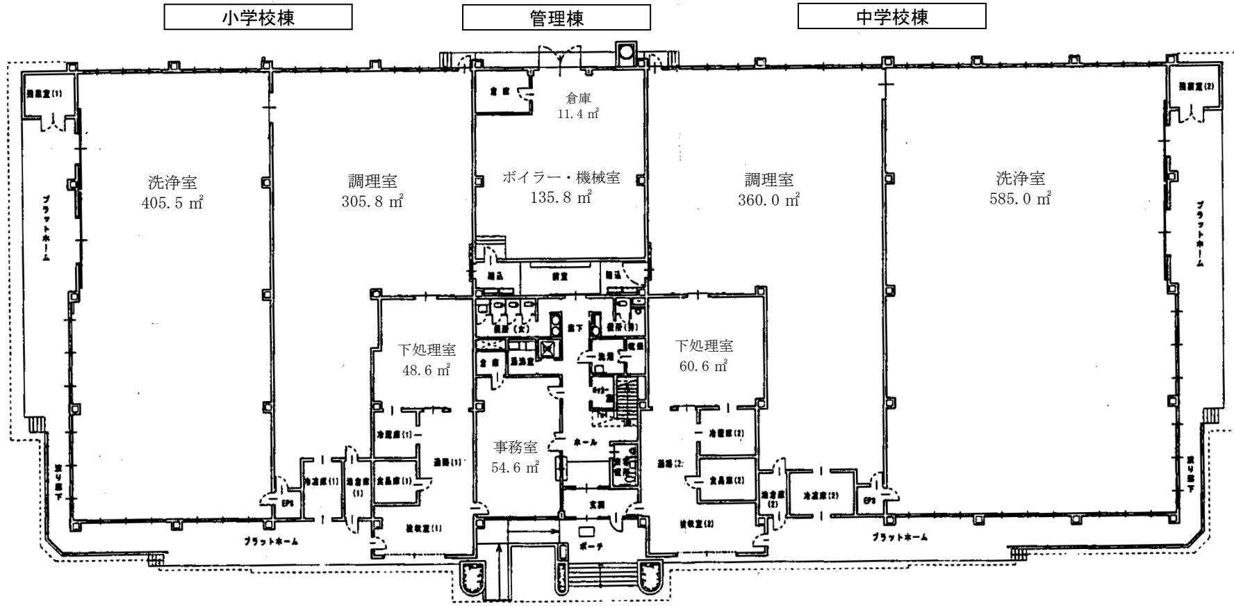
1 階平面図
