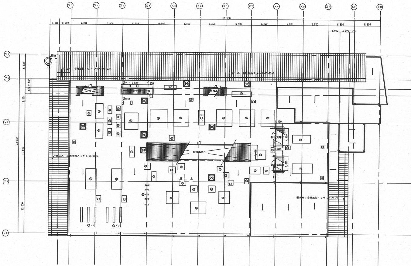
R階平面図 1 : 200
