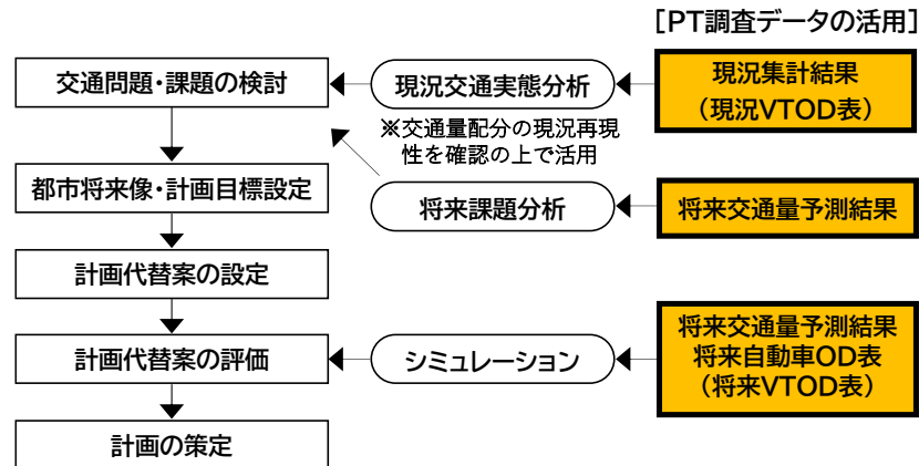
図 7-2 道路網計画の策定手順(例)と使用するPT調査データの関係
