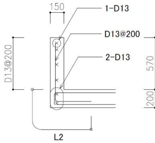
バルコニー端部立上り壁雑詳細図
