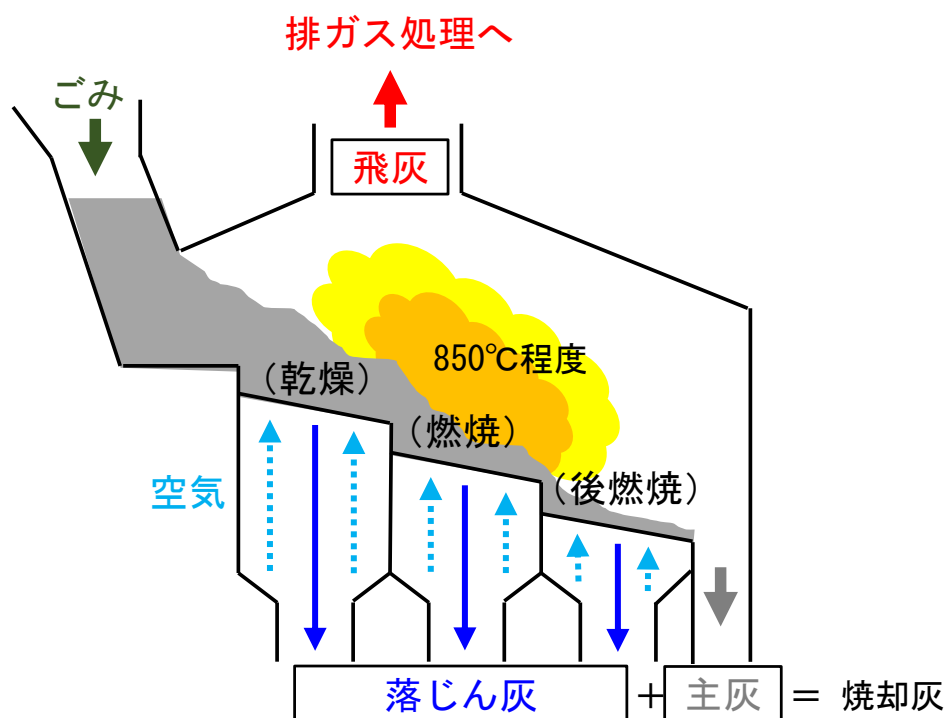
図8-3-1 ストーカ炉における焼却残さ発生図（例）
