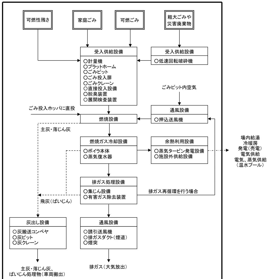
図12-1-1 焼却処理フロー
