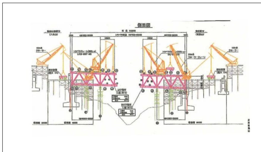
図 5.2.3-2 調査時における施工状況（施工ステップ側面図）平成 24 年 6 月から 7 月
