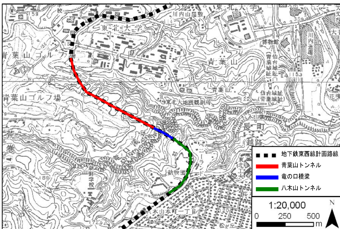
図 5.2.2-3 工事箇所位置図
