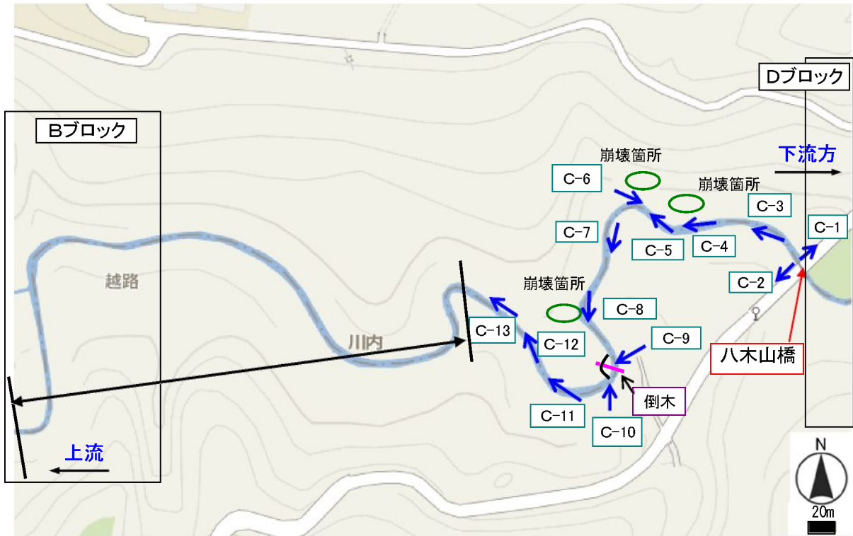
図 5. 2. 2-5(4) 植物調査実施地域（竜の口沢本流沿いの巡回調査：Cブロック写真撮影位置）
