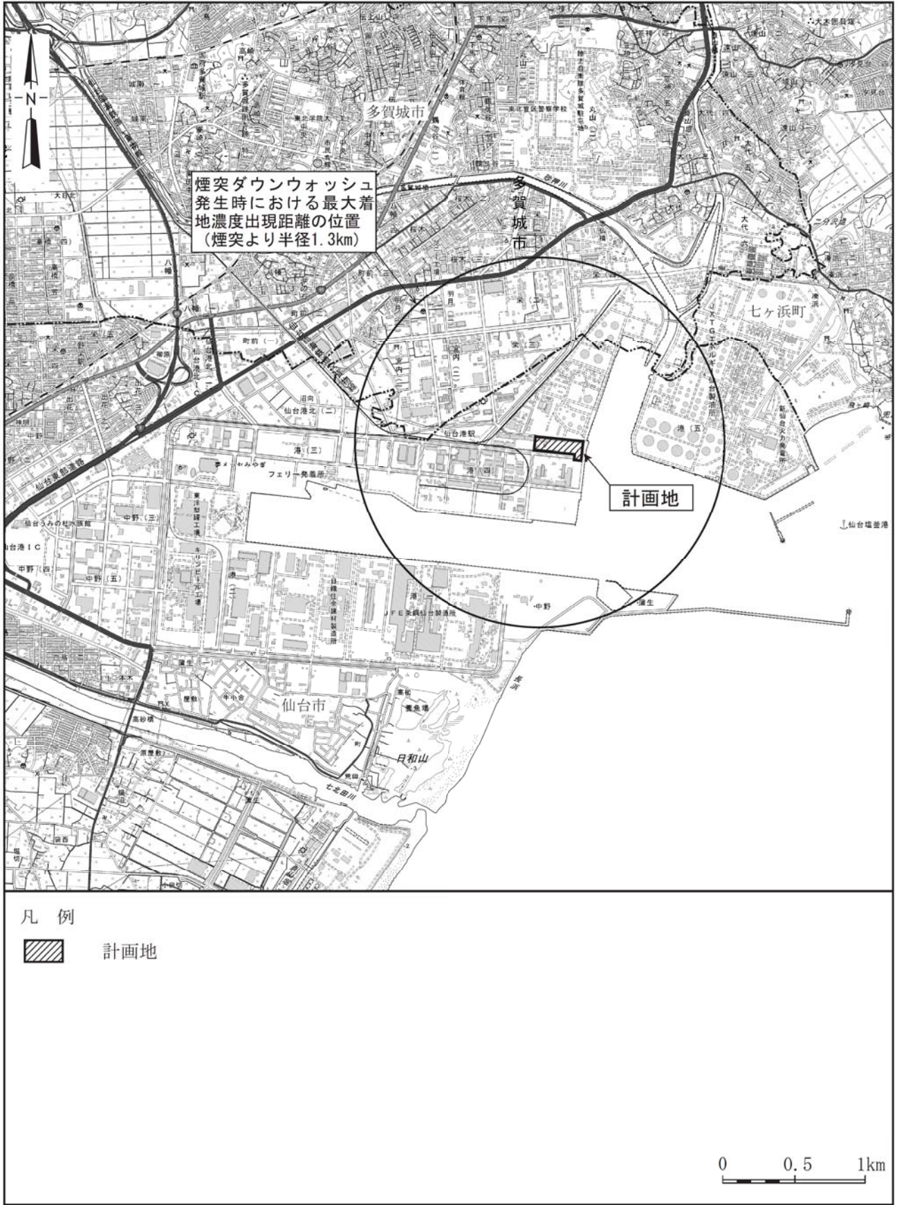
図 8.1-28 最大着地濃度出現距離の位置（煙突ダウンウォッシュ発生時）
