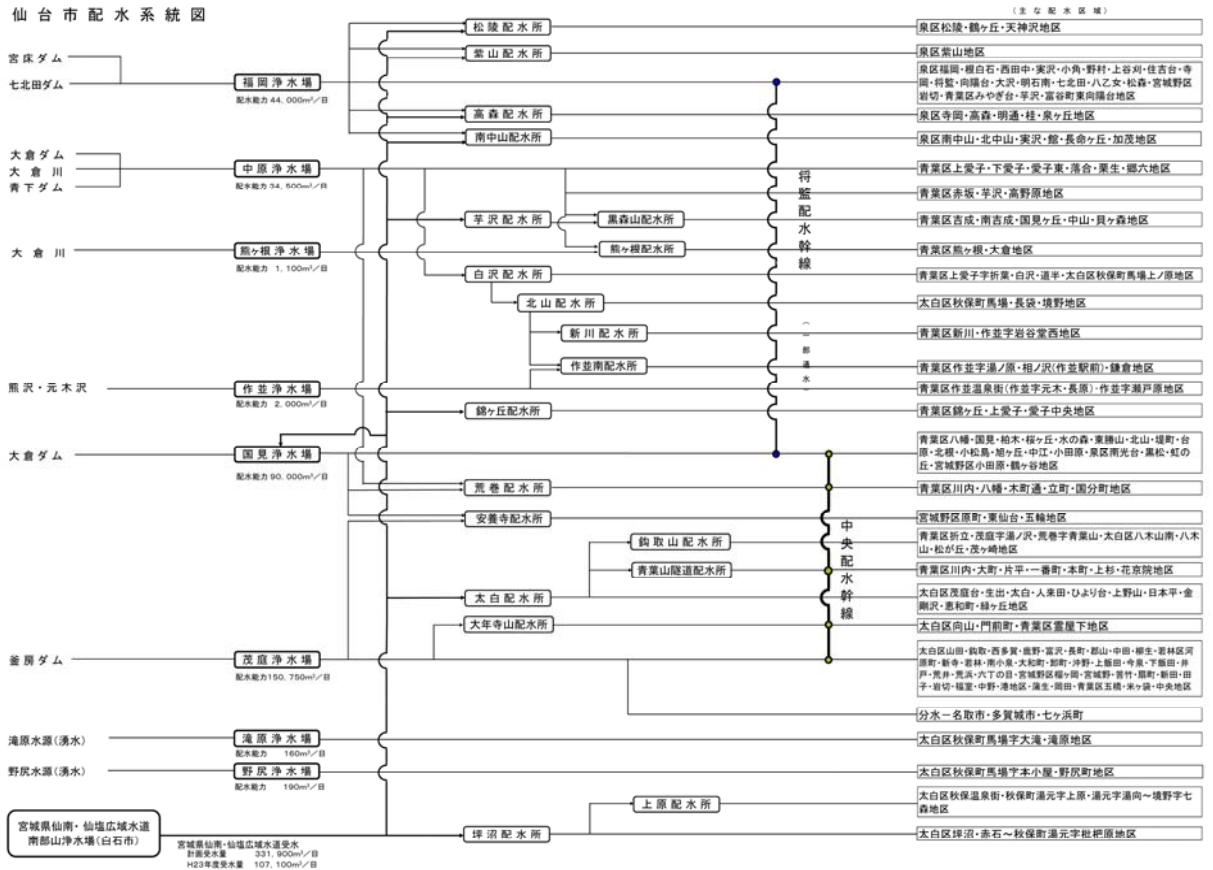
図 3.2-14 配水系統図
