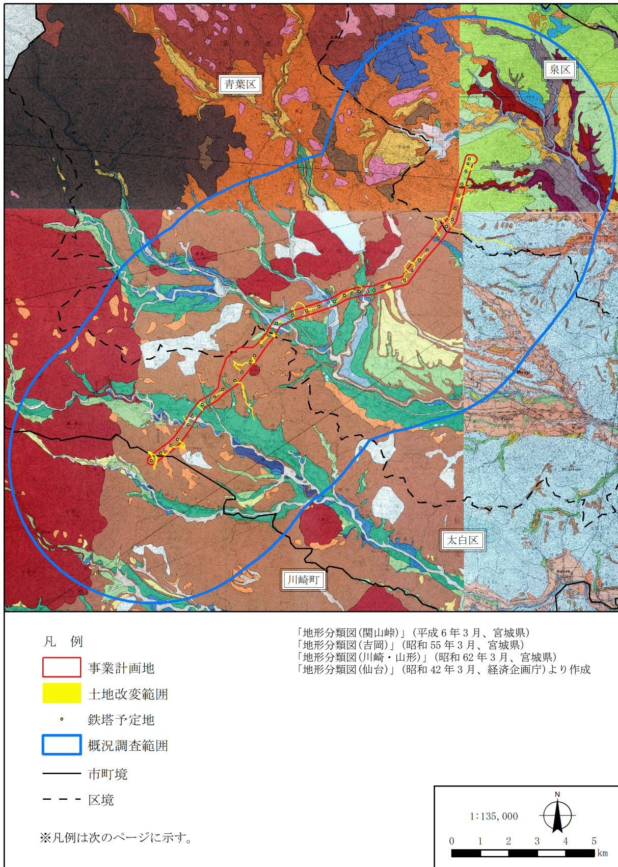
図 6.1.3-1(1) 地形分類
