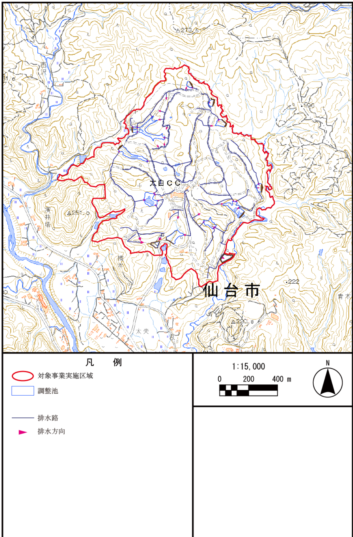
図 2.2-27 雨水排水路の計画図
