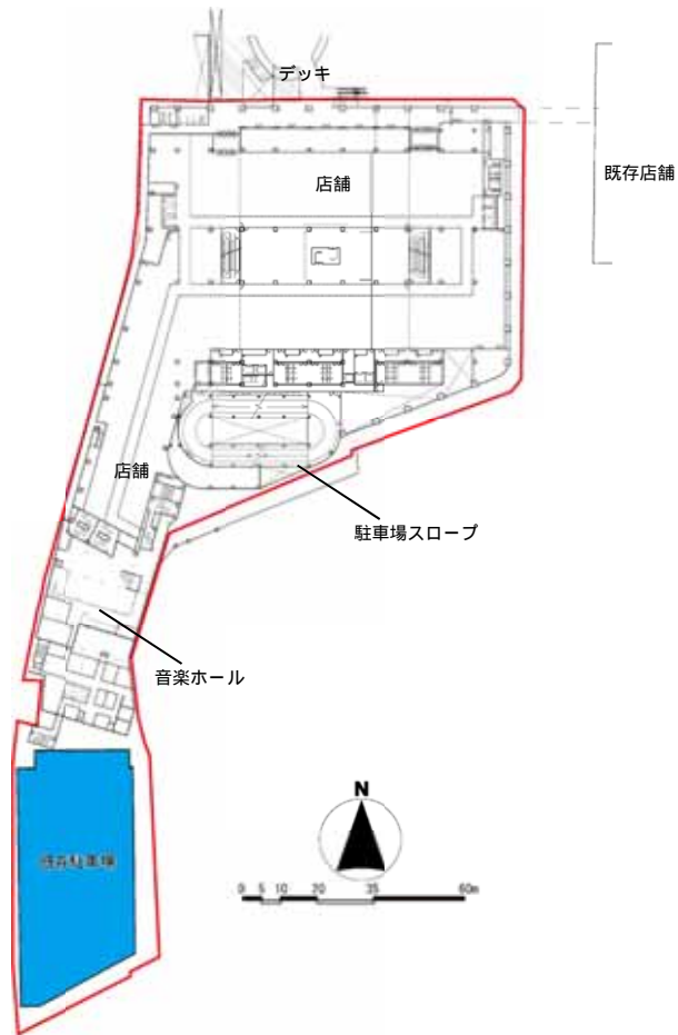
図1-4(5) 各階平面図 ( 3 F )
