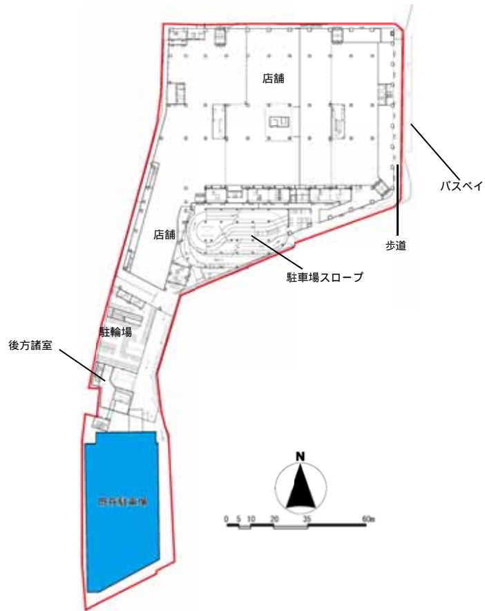
図1-4(3) 各階平面図(1F)
