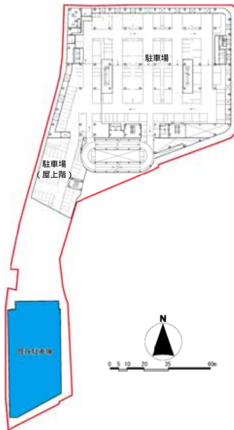
图1-4(10) 各階平面図 ( 8 F )
