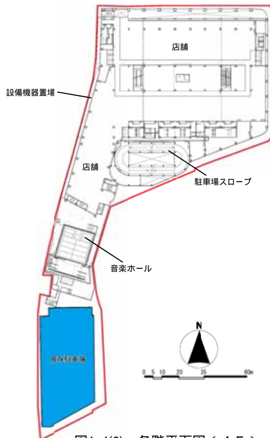
図1-4(6) 各階平面図 ( 4 F )
