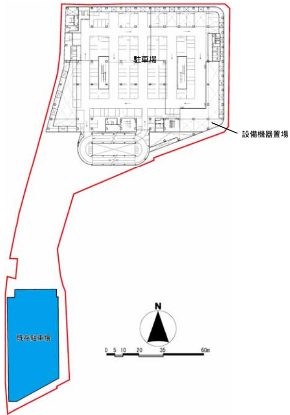
図1-4(11) 各階平面図 ( 9 F )
