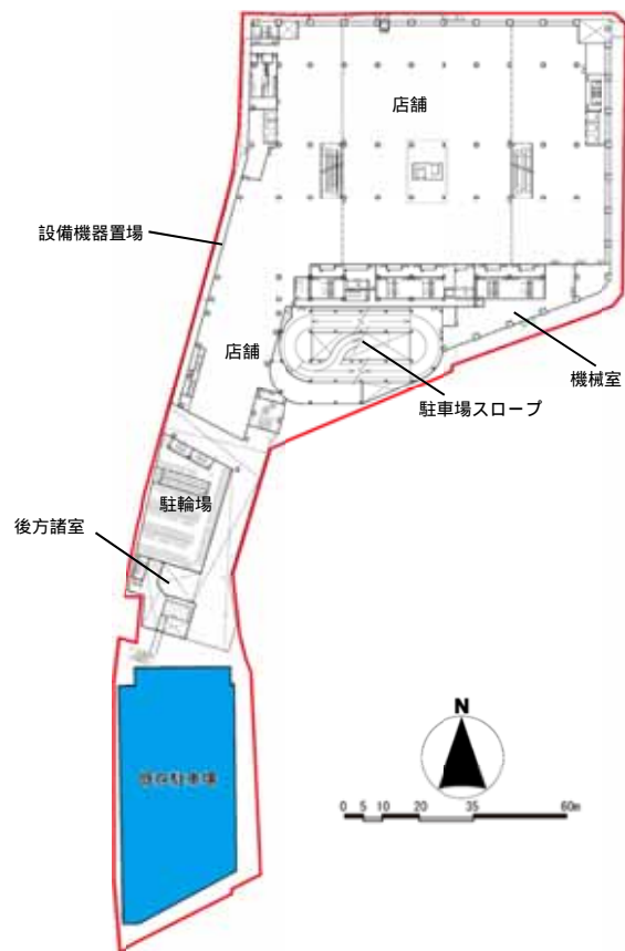
図1-4(4) 各階平面図(2F)
