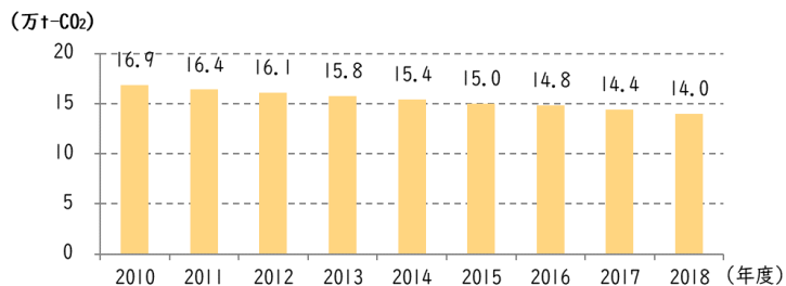
本市における温室効果ガス吸収量の推移
