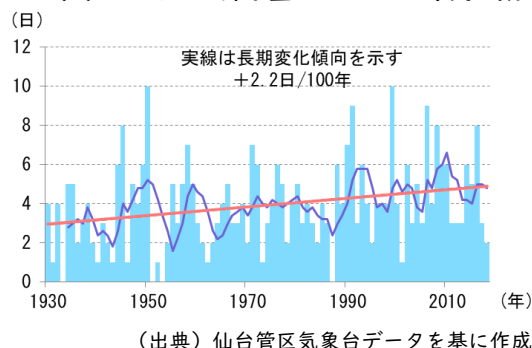
本市における日降水量 50mm 以上の年間日数
