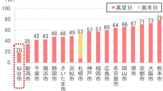
各政令市における真夏日及び真冬日の合計日数
