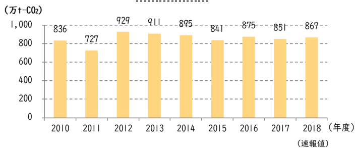
本市における温室効果ガス*排出量の推移
