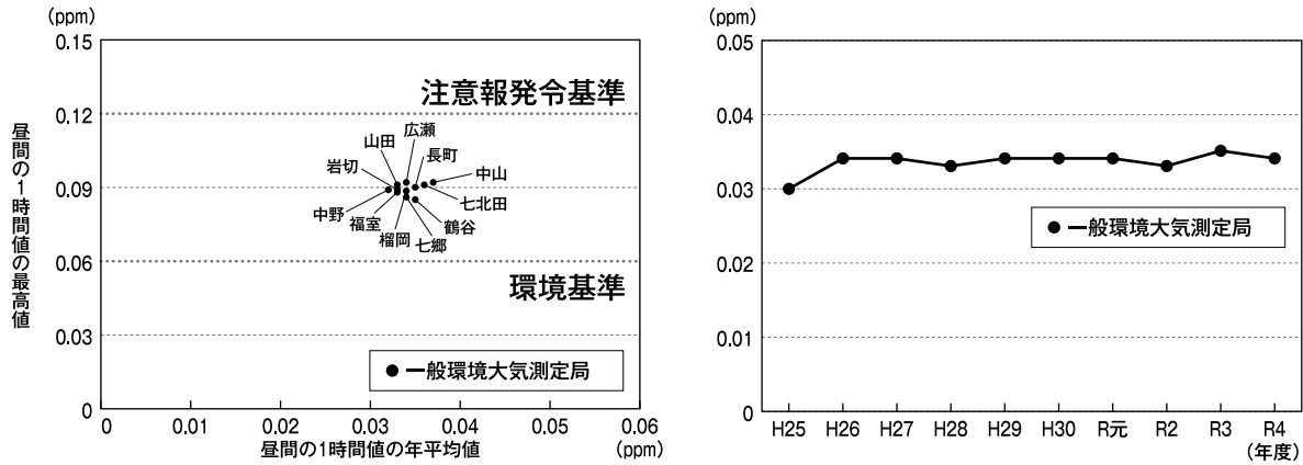
図2-403 光化学オキシダントの測定結果(令和4年度)と昼間の1時間値の年平均値の推移(有効全測定局の平均値)
