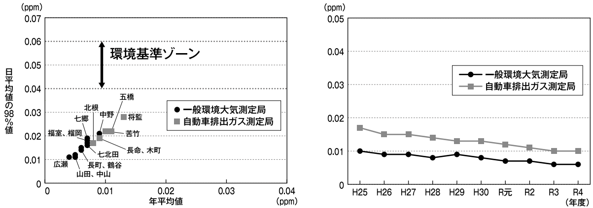
図2-401 二酸化窒素の測定結果(令和4年度)と年平均値の推移(有効全測定局の平均値)
