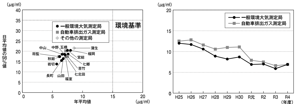
図2-402 微小粒子状物質の測定結果(令和4年度)と年平均値の推移(有効全測定局の平均値)
