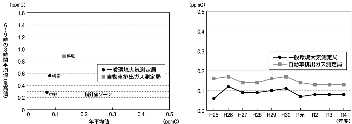
図2-404 非メタン炭化水素の測定結果(令和4年度)と年平均値の推移(有効全測定局の平均値)
