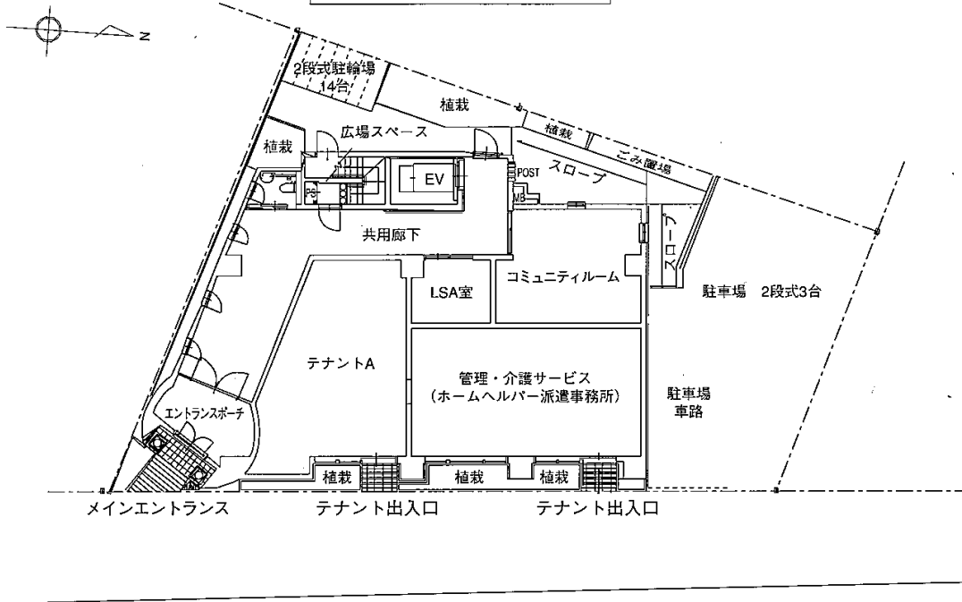
配置図・1階平面図
