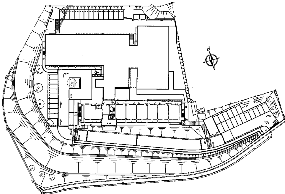
敷地配置図
