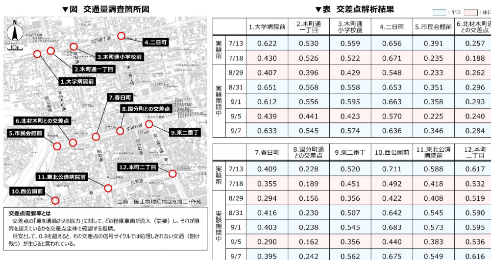
図 交差点解析結果（交差点需要率）
