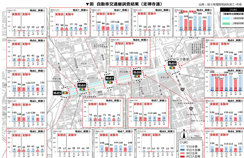
図 0-1 自動車交通量調査結果（定禅寺通）
