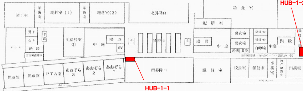
○ 1F平面図
