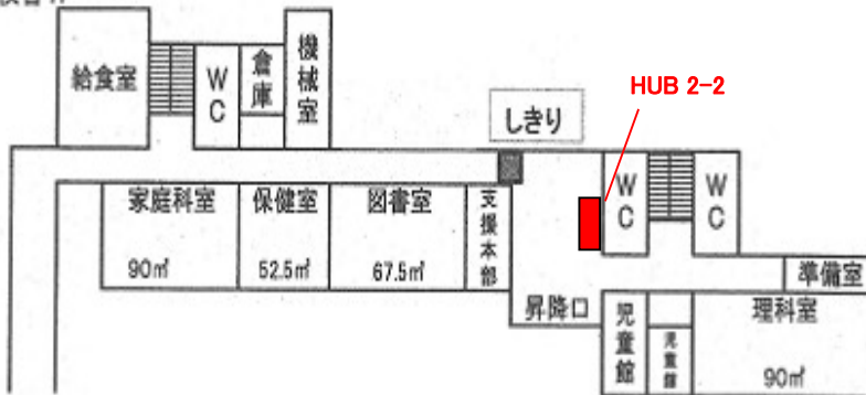
北校舎1F
